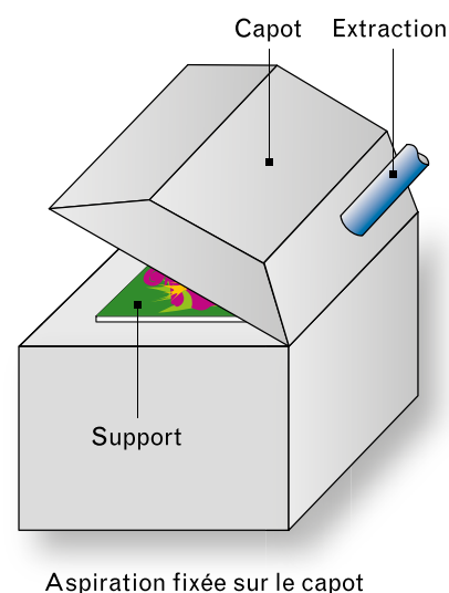
Figure 6. Différents dispositifs de captage pour machine de sérigraphie.
