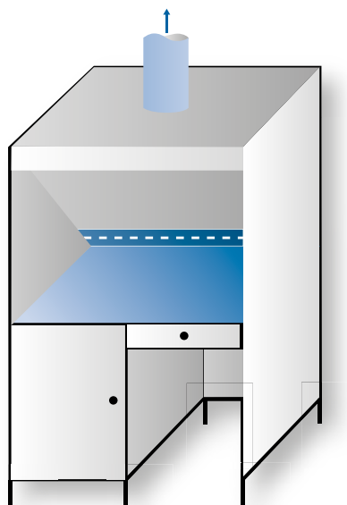
Figure 5. Schéma d'un poste de préparation des encres, valable également pour la préparation des écrans.
